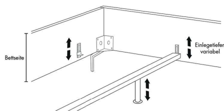
Einlegetiefen
